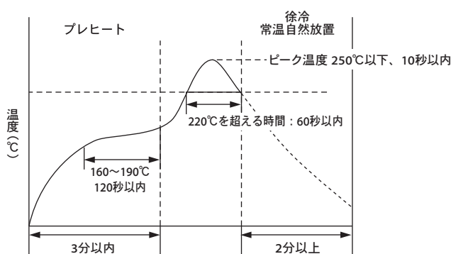
はんだ付け温度プロファイル (リフロー)
